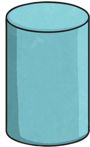
silindr
