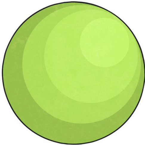
sffêr
