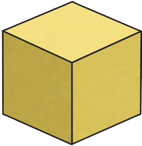
ciwb
