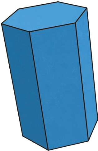
prism hecsagonol
