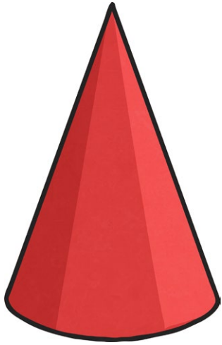
côn
